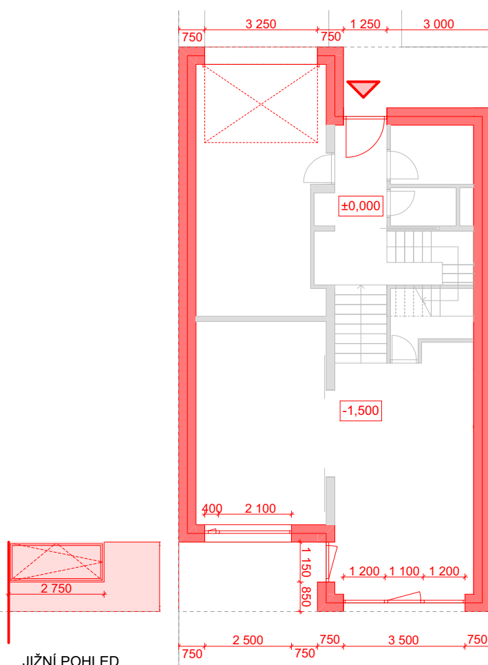
JIŽNÍ POHLED
