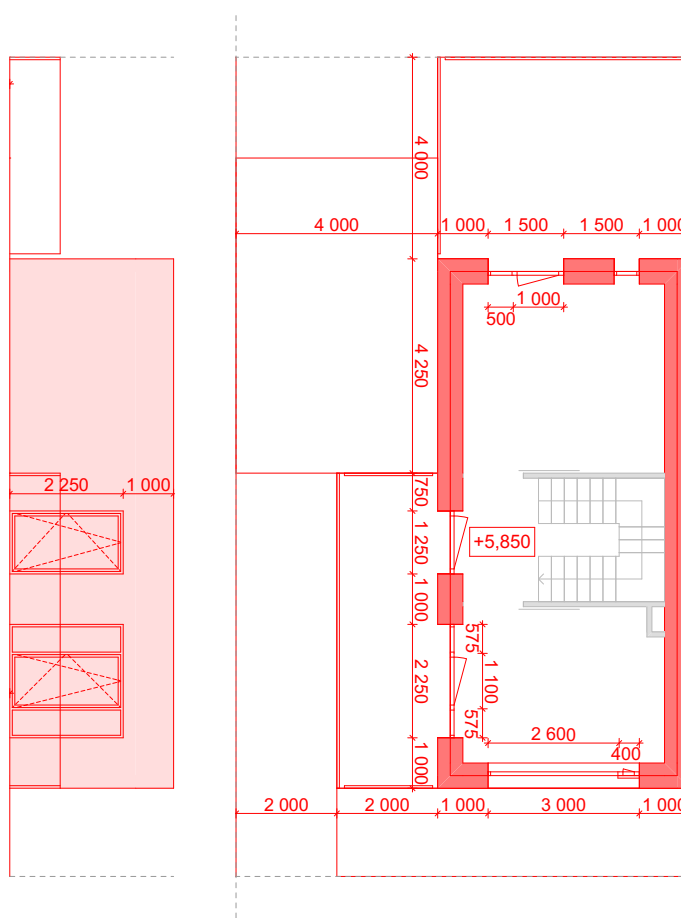
JIŽNÍ POHLED
