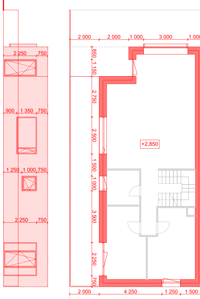
JIŽNÍ POHLED
