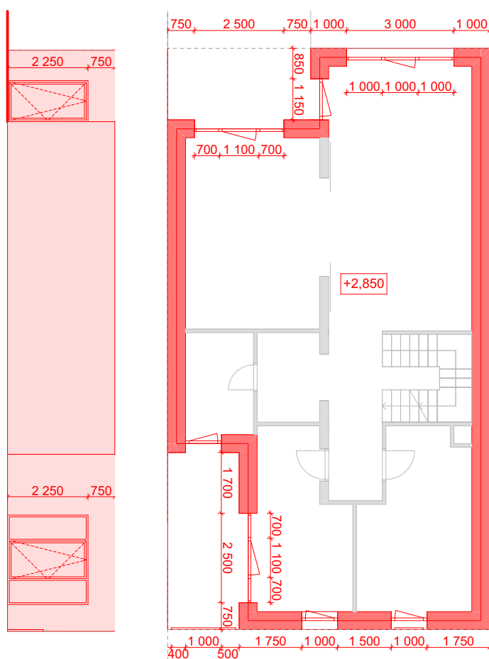
JIŽNÍ POHLED
