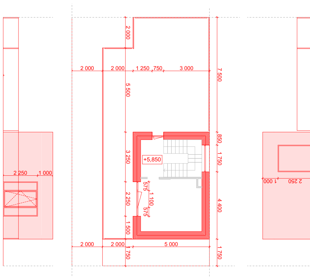
JIŽNÍ POHLED
