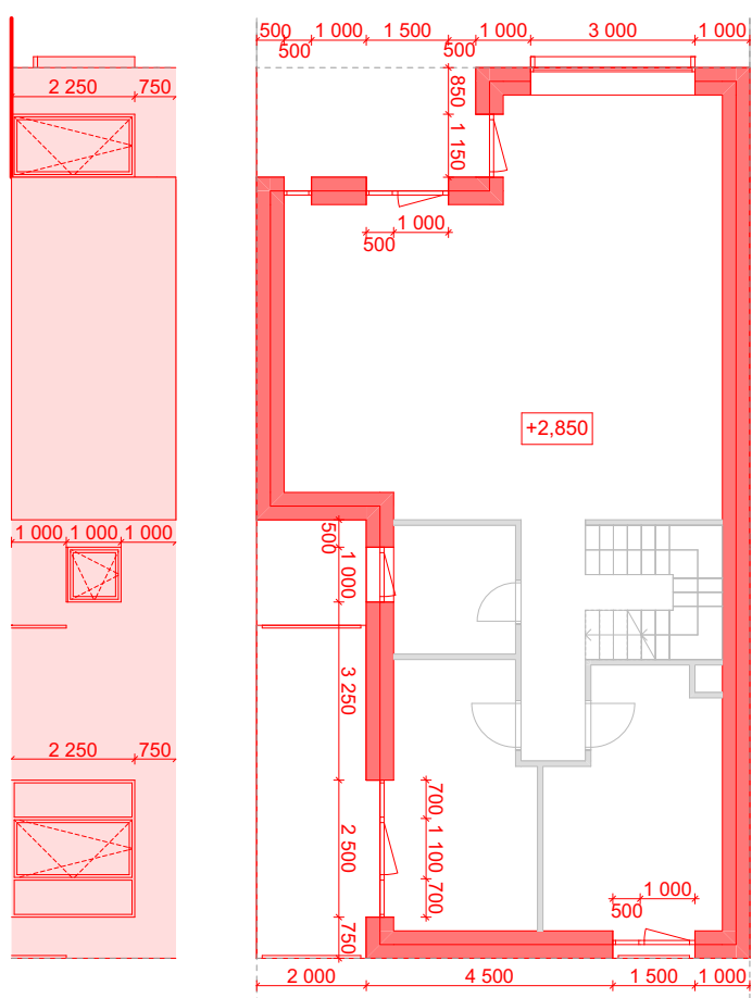
JIŽNÍ POHLED
