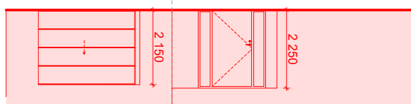
SEVERNÍ POHLED - Z ULICE
