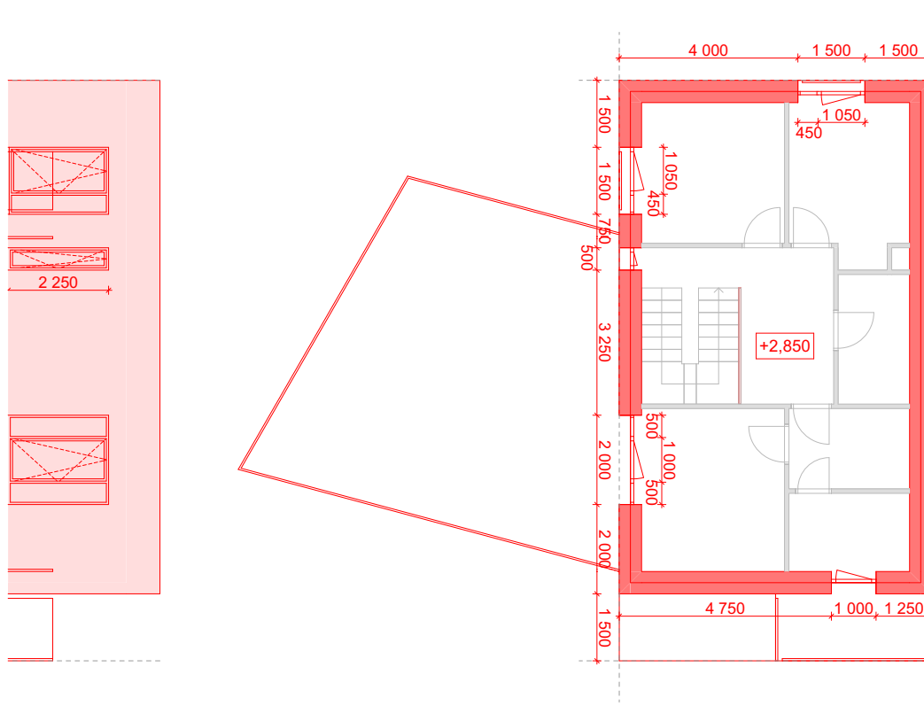
ZÁPADNÍ POHLED
