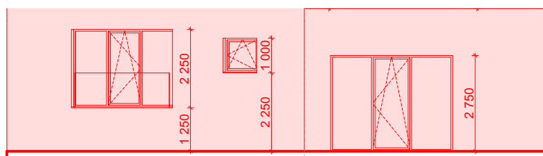
JIŽNÍ POHLED - ZE ZAHRADY
